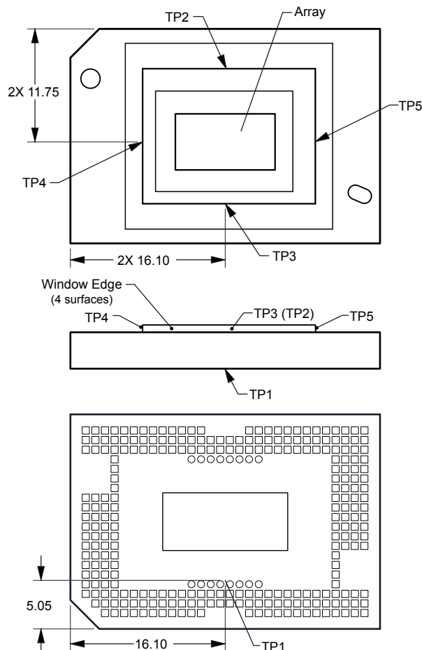
図 6-2. DMD Thermal Test Points
