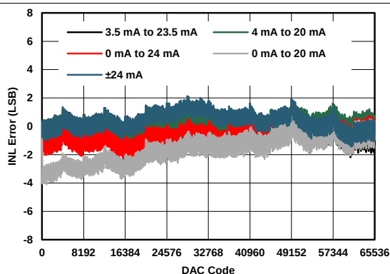
図 3. IOUT Linearity Error vs Digital Input Code
