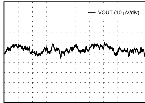
图 27. VOUT Noise (DC/DC Disabled)
