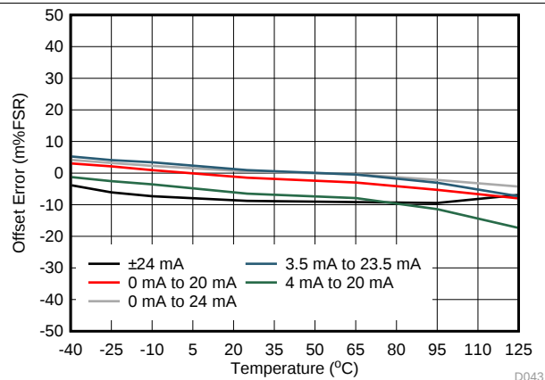
图 47. IOUT Offset Error vs Temperature
