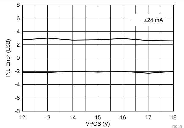
图 49. IOUT Bipolar Range INL vs VPOS
