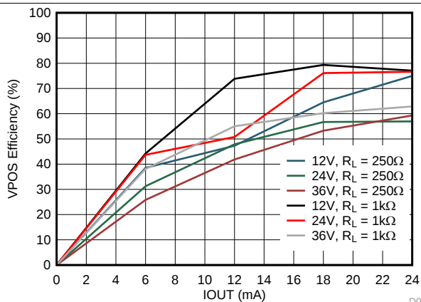
图 79. IOOUT VPOS Efficiency
