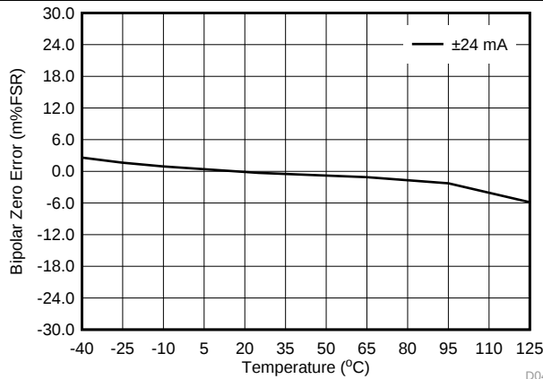
图 44. IOUT Bipolar Zero Error vs Temperature
