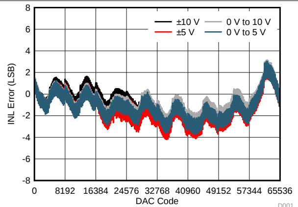
図 4. VOUT INL vs Code (DC/DC Enabled)
