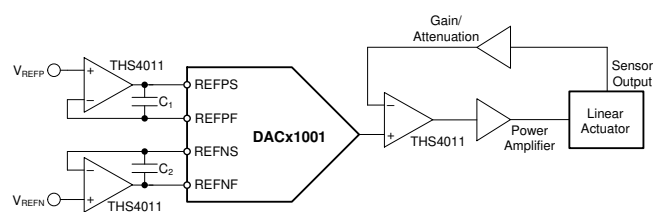
高精度の制御ループ回路
