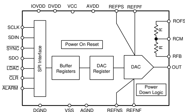
機能ブロック図
