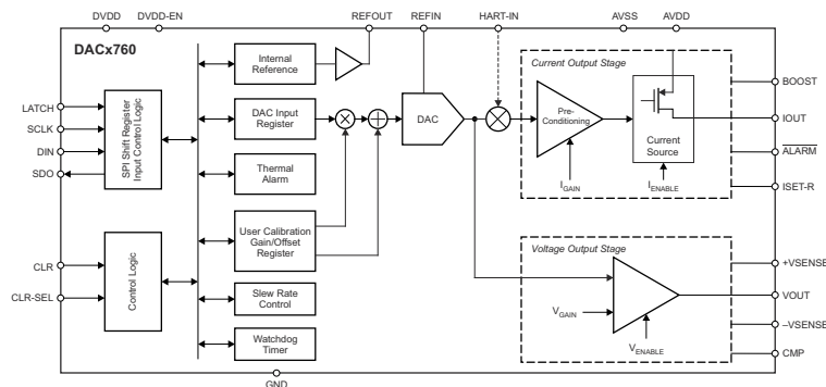
ブロック図
