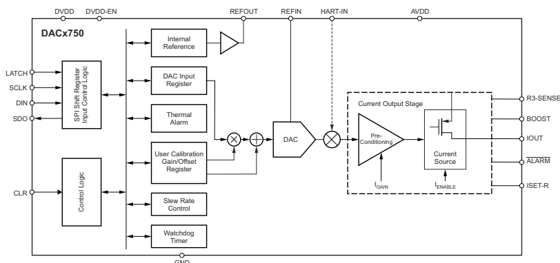
ブロック図
