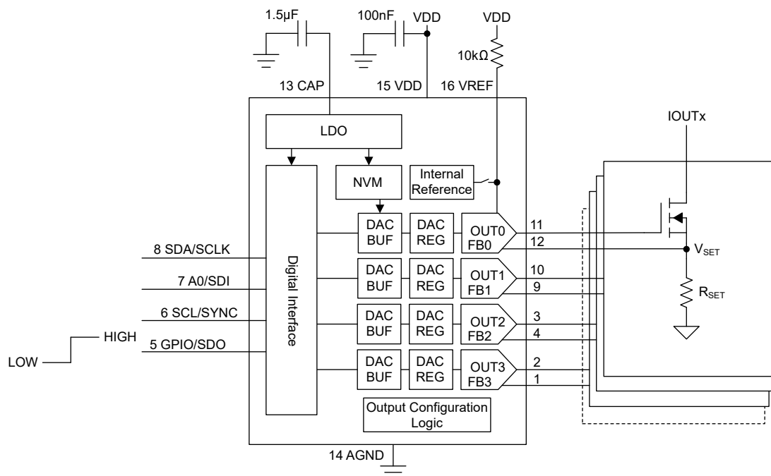
図 8-1. Current Source
