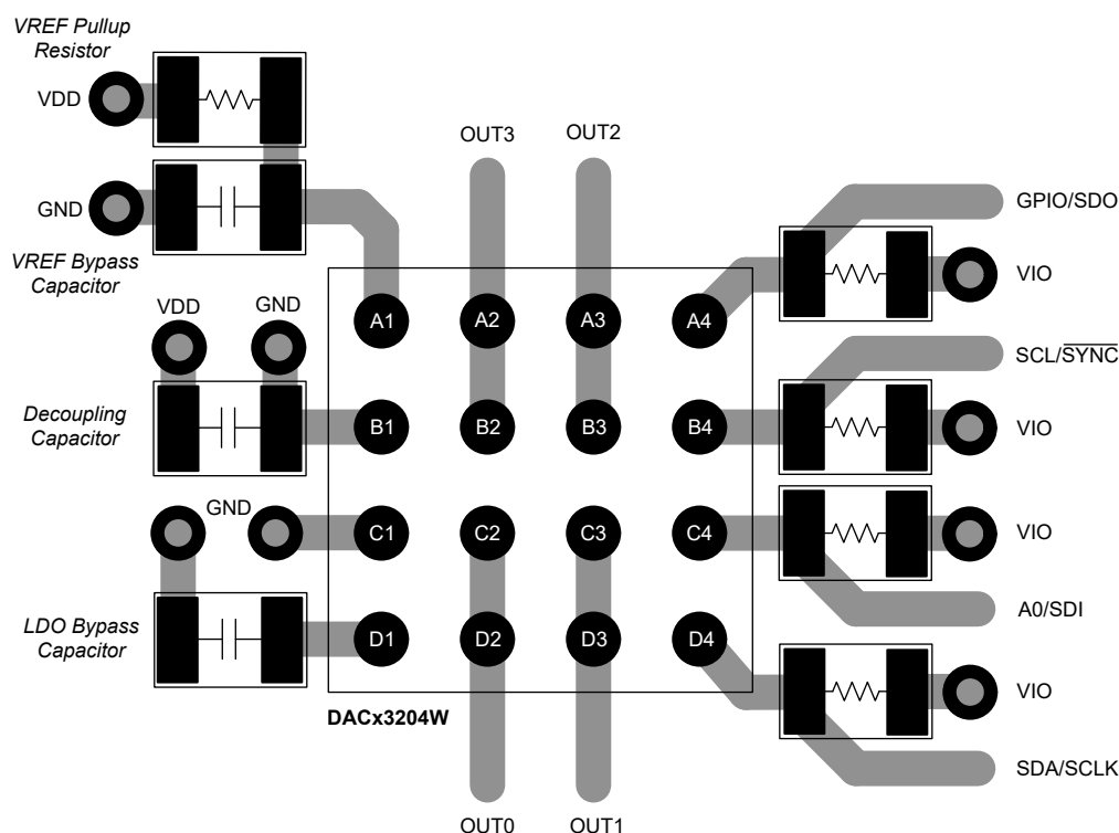
图 8-3. Layout Example
