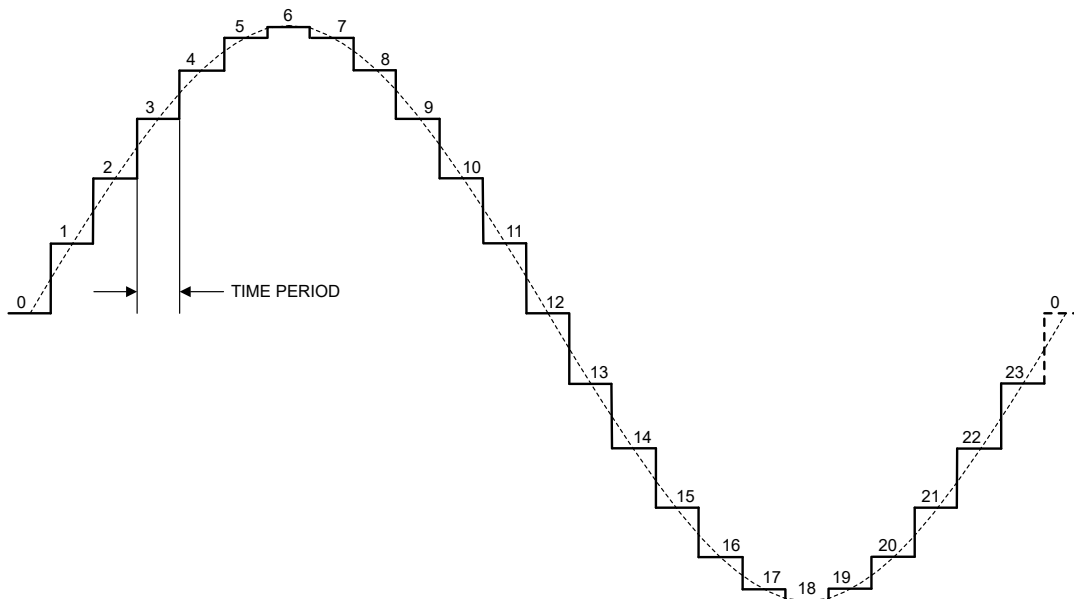
図 7-14. Sine Wave Generation
