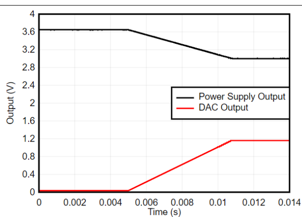
図 8-3. Power-Supply Margin Low
