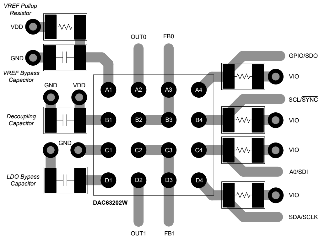
图 8-4. Layout Example
