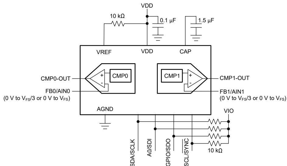
図 7-3. Comparator Interface
