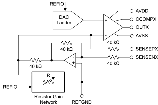
図 8-3. Voltage Output Buffer
