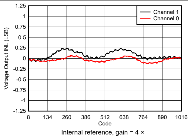
图 6-4. Voltage Output INL vs Digital Input Code
