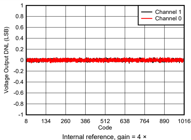
图 6-8. Voltage Output DNL vs Digital Input Code
