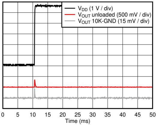
图 40. Power-on Glitch
