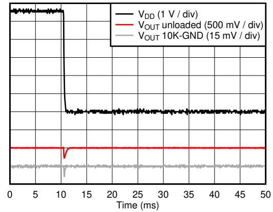
图 41. Power-off Glitch
