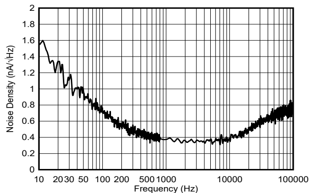
图 6-49. Current Output Noise Density
