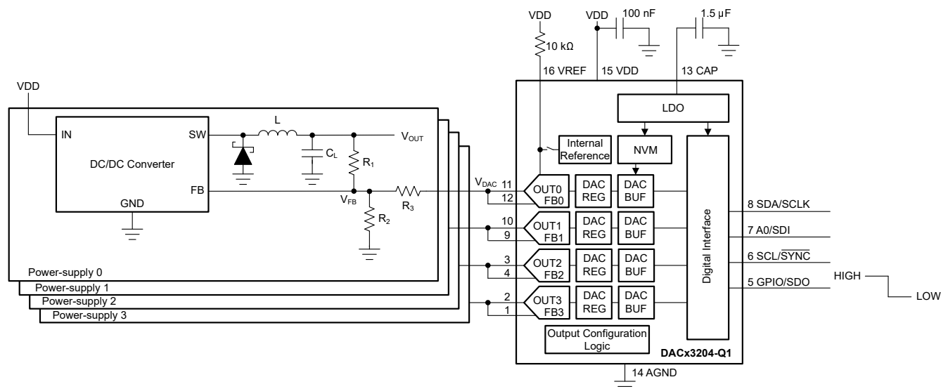
図 8-1. APD Biasing
