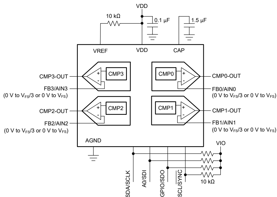
図 7-3. Comparator Interface
