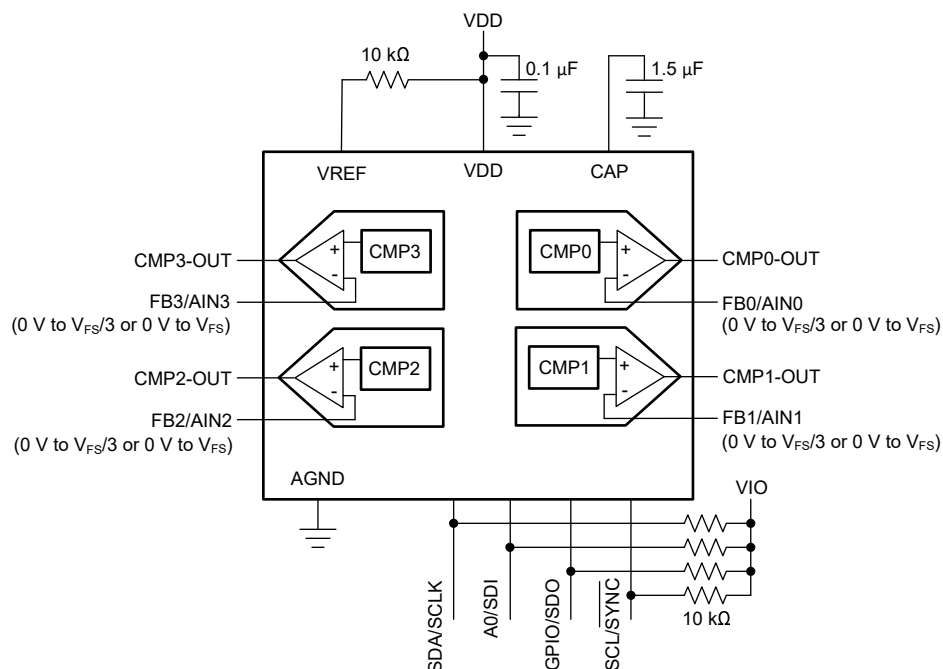
图 7-3. Comparator Interface
