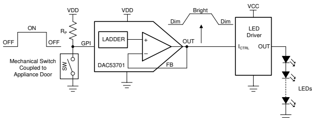
家電製品のライト・フェードイン・フェードアウト
