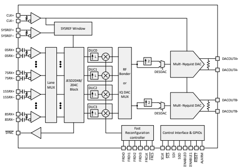
ブロック図
