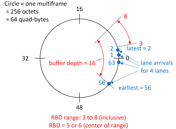
FIG 7-56. RBD Example (lane arrivals straddle zero)
