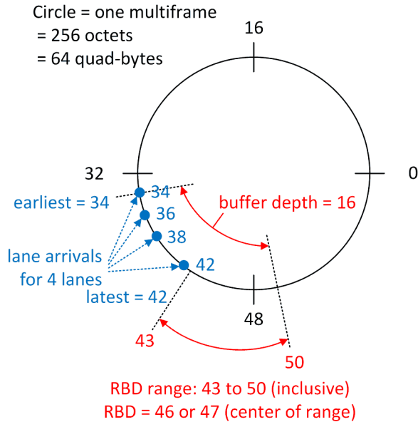
FIG 7-55. RBD Example (lane arrivals do not straddle zero)
