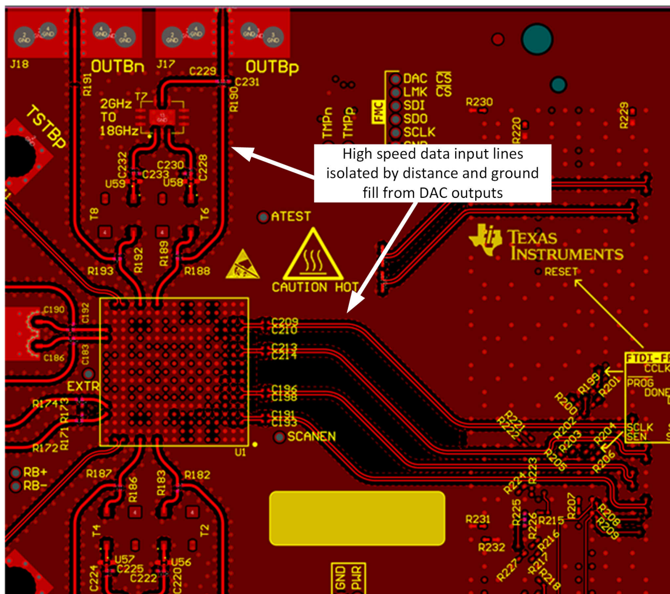
図 9-13. グランドフィル絶縁による Serdes の上層配線
