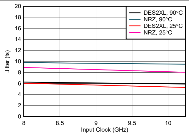
图 6-221. Jitter vs Input Clock
