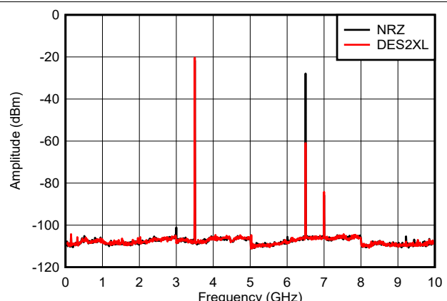
✎ 6-28. f_{\text{OUT}} = 3497\text{ MHz} , 0dBFS
