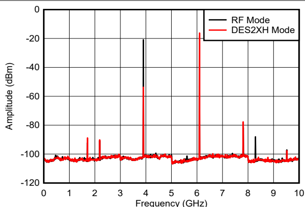
図 6-32. f_{\text{OUT}} = 6097\text{MHz} , -6dBFS
