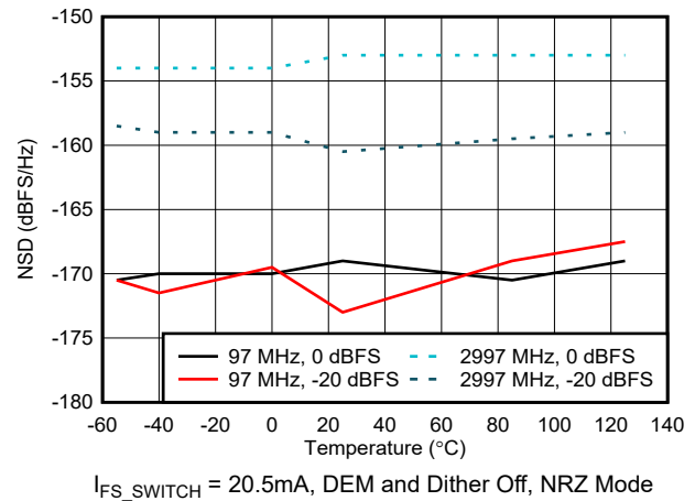
図 6-81. NSD vs Temperature
