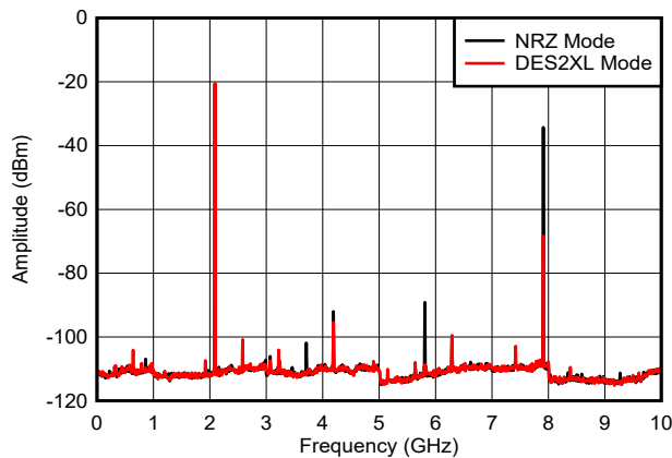
✎ 6-25. f_{\text{OUT}} = 2097\text{ MHz} , 0dBFS
