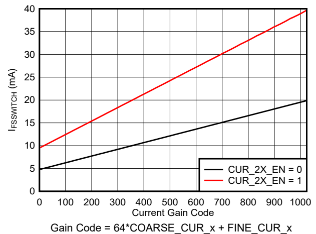
図 6-15. I_{\text{FS\_SWITCH}} vs Gain Code
