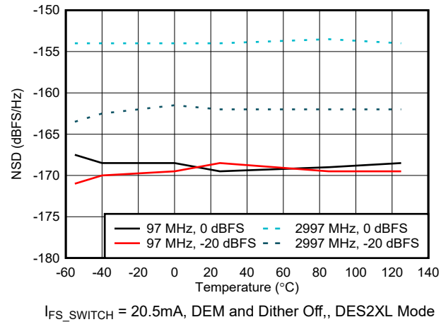
図 6-83. NSD vs Temperature
