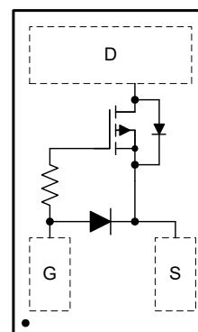
図 3-2. 上面図
