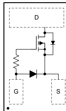
上面図
