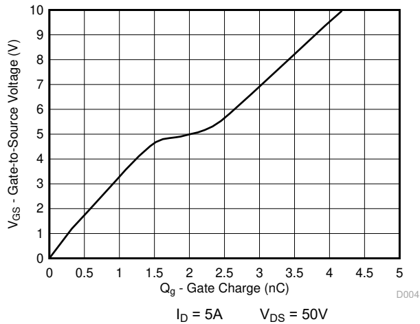
図 3-4. Gate Charge
