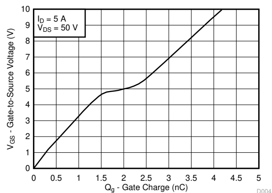
ゲート電荷
