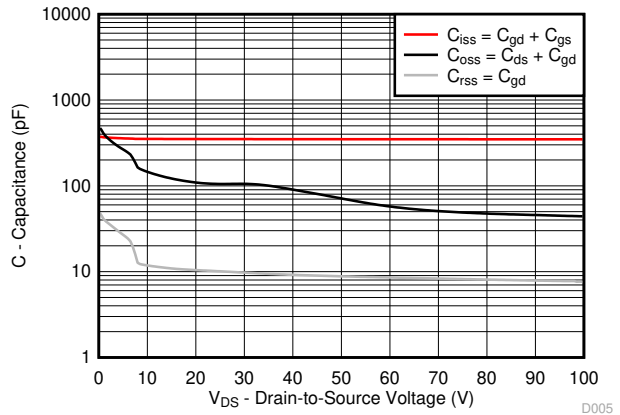
図 3-5. Capacitance
