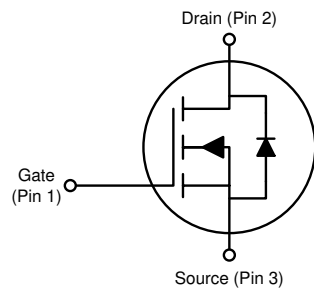
ピン配置
