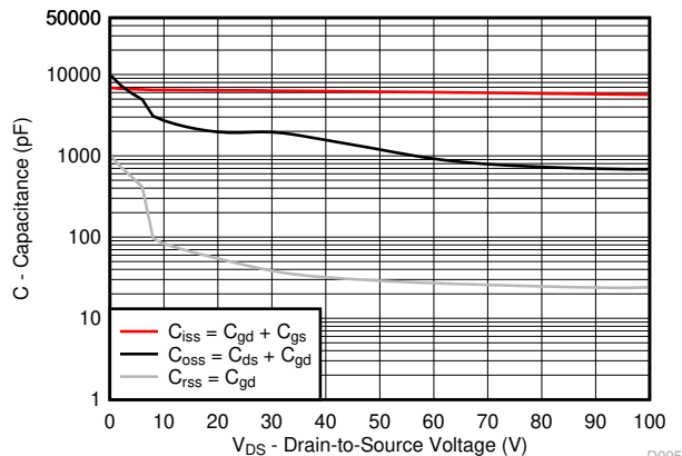
図 4-5. 容量
