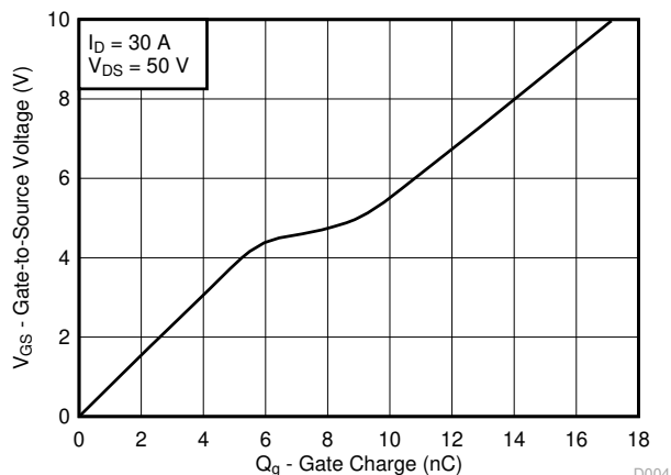
ゲート電荷
