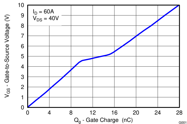
ゲート電荷
