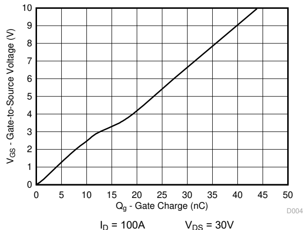
図 4-4. Gate Charge
