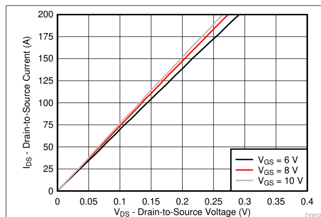
図 4-2. 飽和特性
