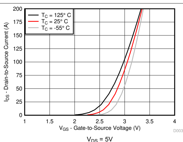
図 4-3. 伝達特性
