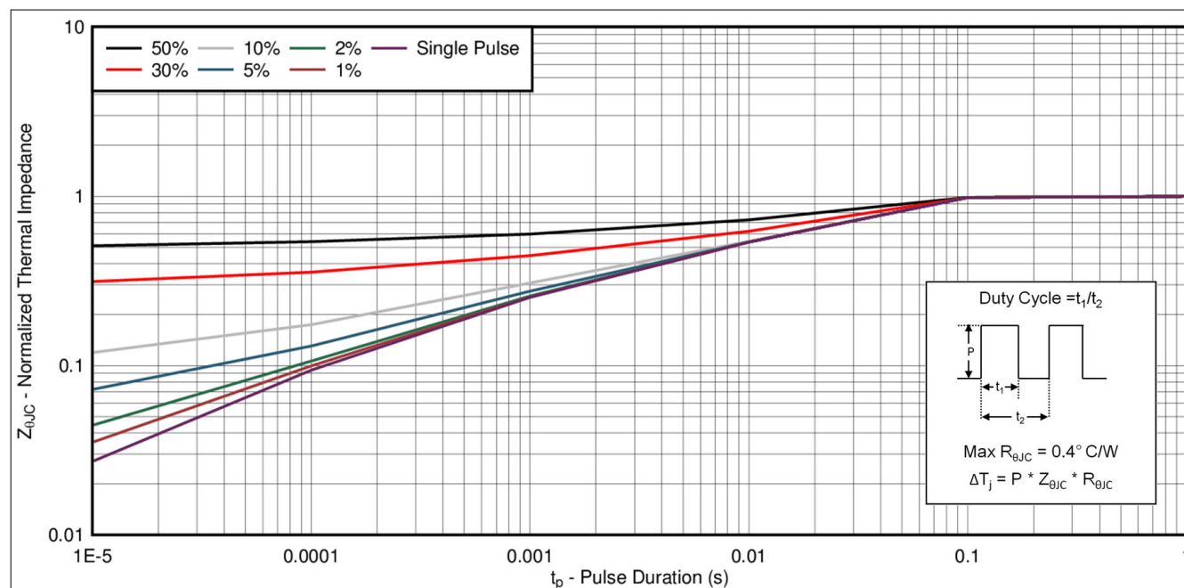
図 4-1. 過渡熱抵抗
