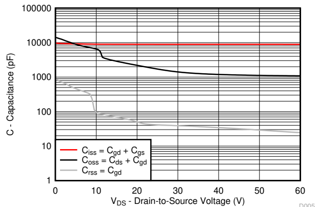
図 4-5. 容量
