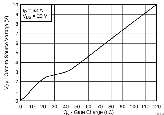
ゲート電荷
