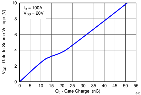
図 4-4. Gate Charge
