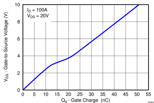
ゲート電荷
