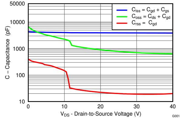
図 4-5. Capacitance
