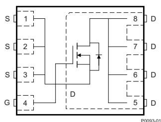
上面図
