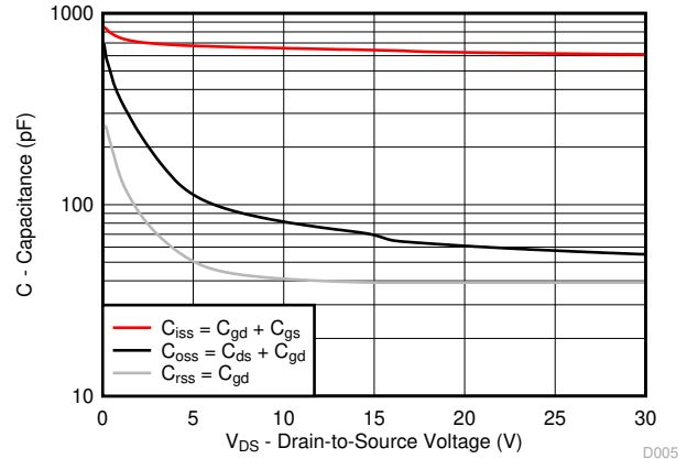
図 4-5. Capacitance
