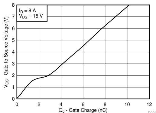
ゲート電荷
