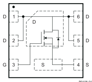
図 3-1. 上面図
