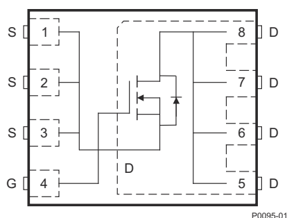
上面図
