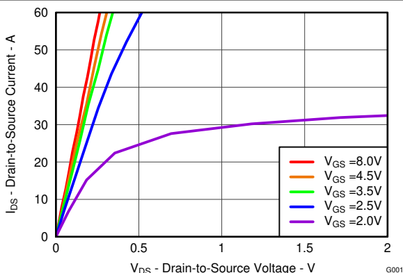
図 5-2. 飽和特性
