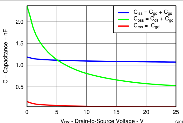
図 5-5. 容量
