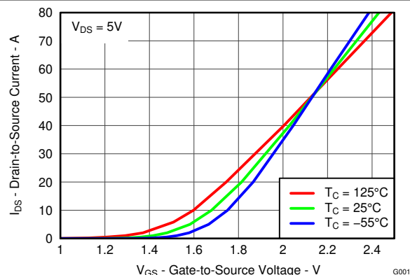
図 5-3. 伝達特性
