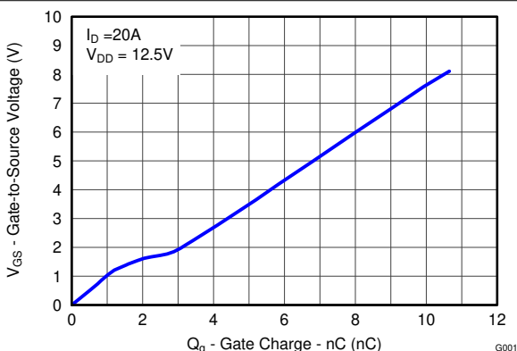
図 5-4. ゲート電荷
