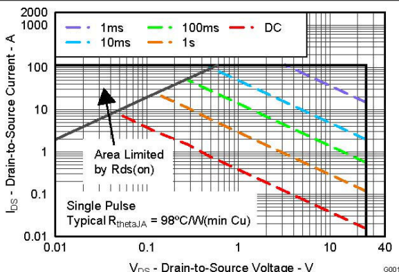
図 5-10. 安全動作領域 (最大値)
