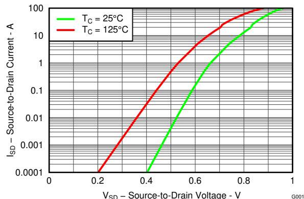
図 5-9. ダイオードの順方向電圧 (標準値)
