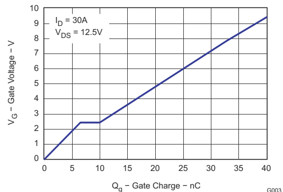
ゲート電荷
