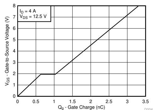
ゲート電荷
