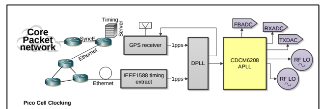
概略回路図
