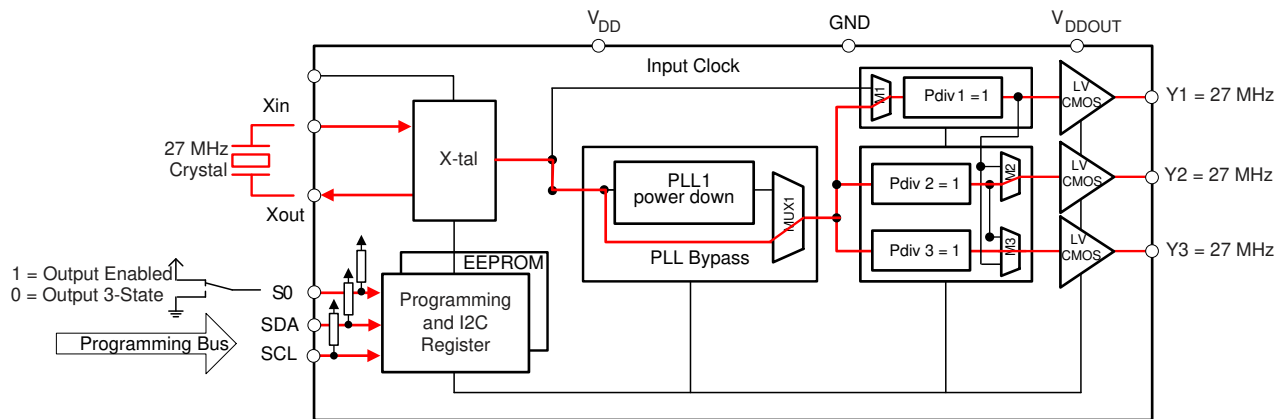
図 8-1. Default Configuration
