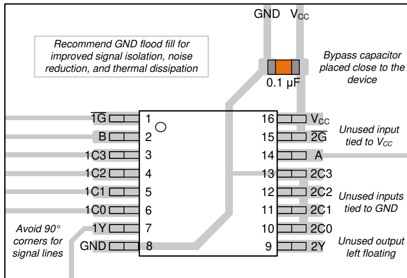
図 7-1. CD74AC153 のレイアウト例
