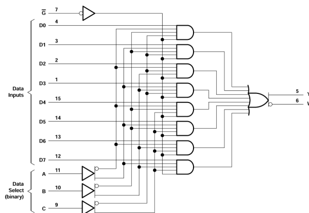
論理図 (正論理)
