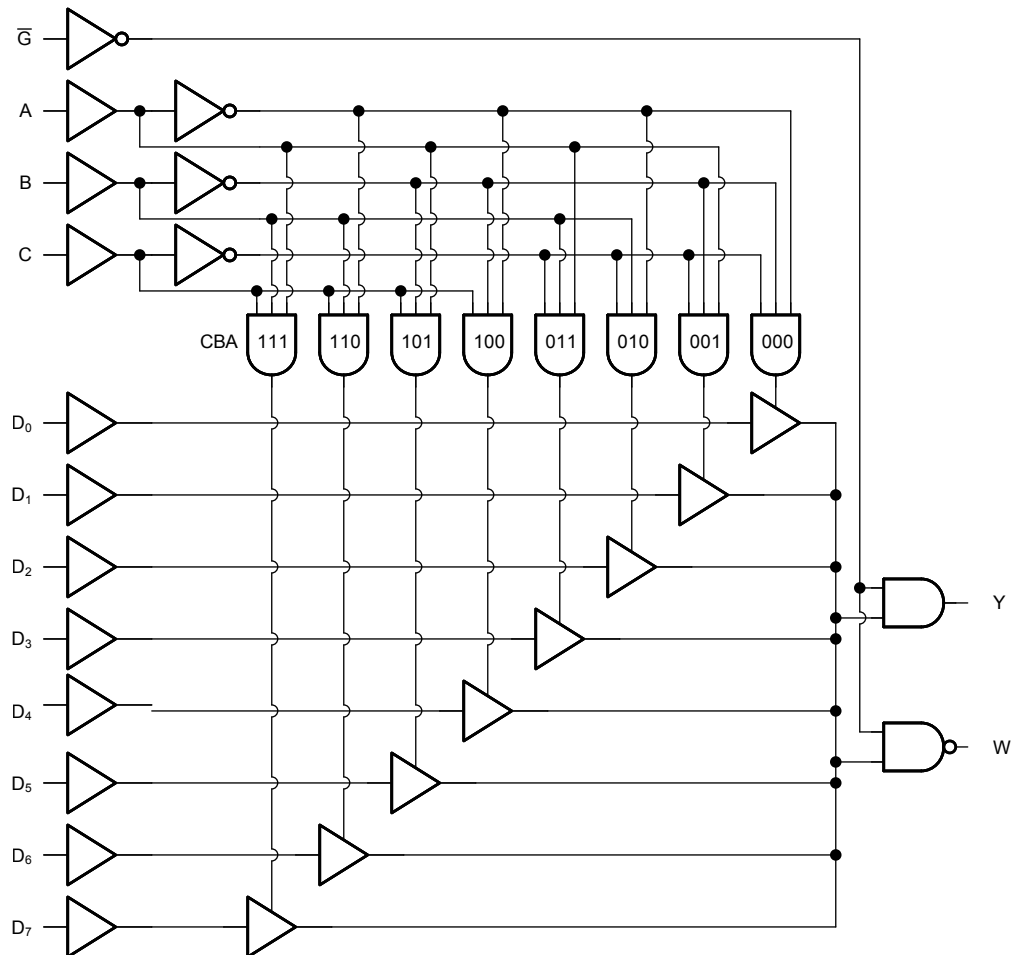
図 6-1. CDx4ACT151 の論理図 (正論理)
