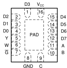
図 3-2. CD74ACT151 BQB パッケージ、16 ピン WQFN (透過上面図)
