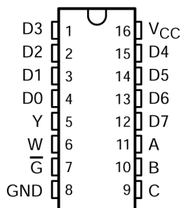
図 3-1. CD54ACT151 J パッケージ、CD74ACT151 J、D、または PW パッケージ、16 ピン CDIP、SOIC、または TSSOP (上面図)
