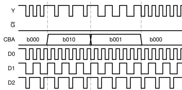
図 7-2. アプリケーション タイミング図
