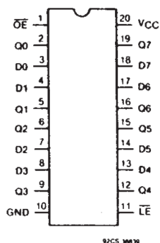
図 3-1. CDx4AC373, CDx4ACT373
