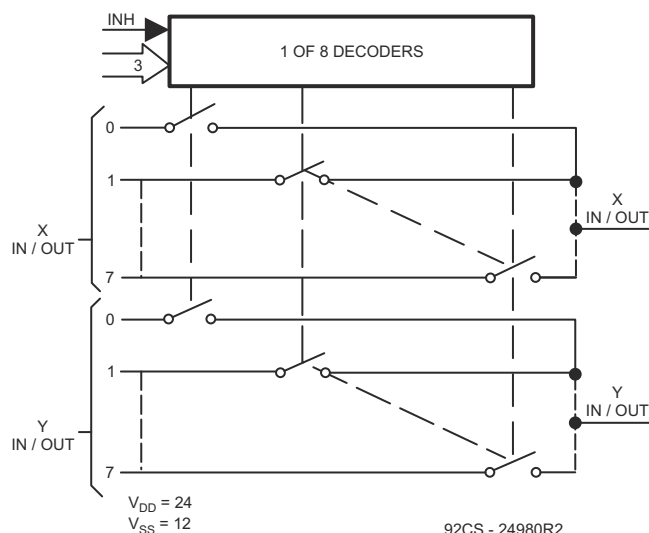
图 7-2. CD4097
