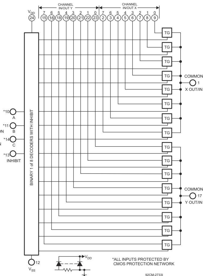
CD4097 の論理図
