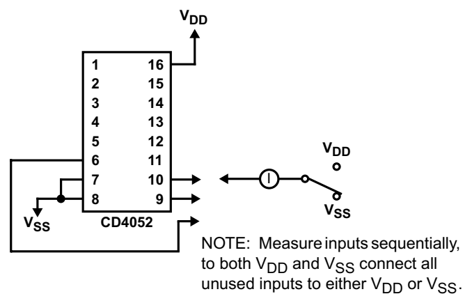
図 6-12. Input Current
