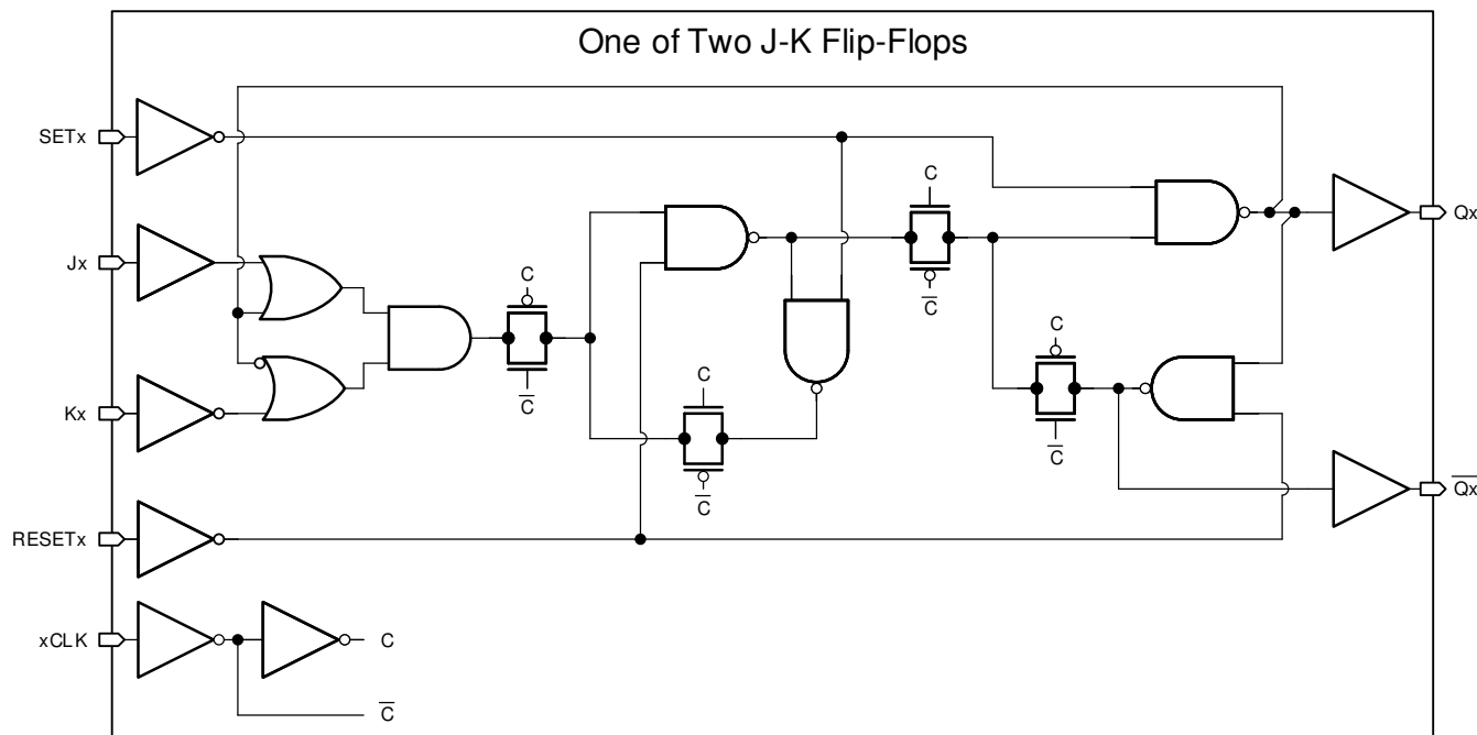
図 3-1. ロジック図
