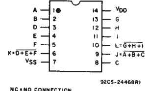
CD4025B
