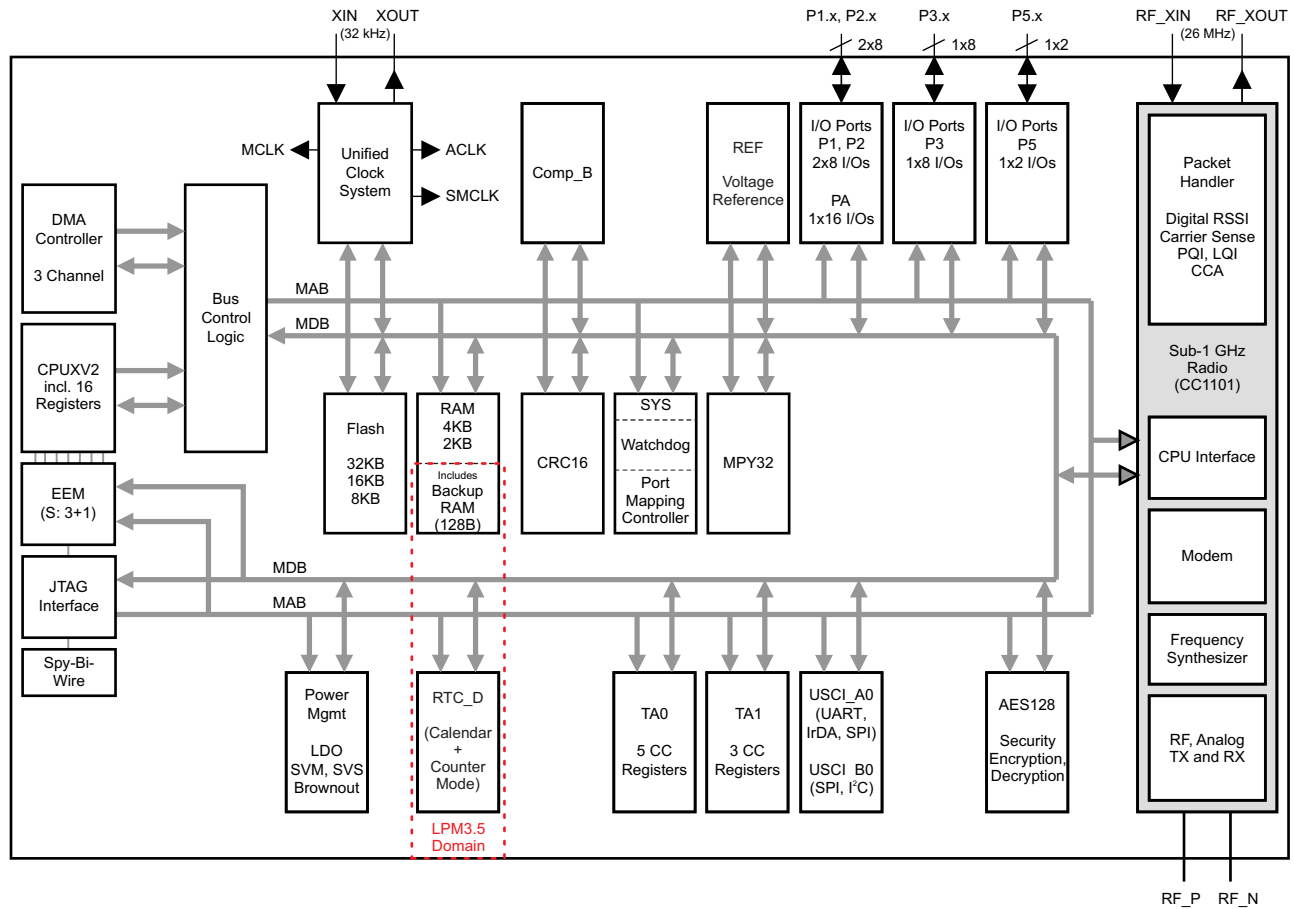
図 1-3. CC430F512xの機能ブロック図
