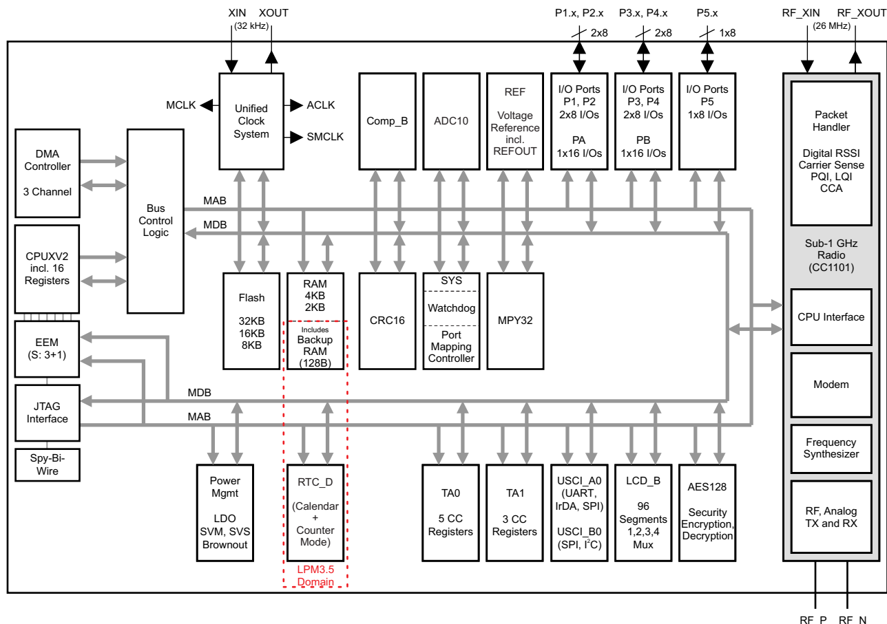
図 1-1. CC430F614xの機能ブロック図
