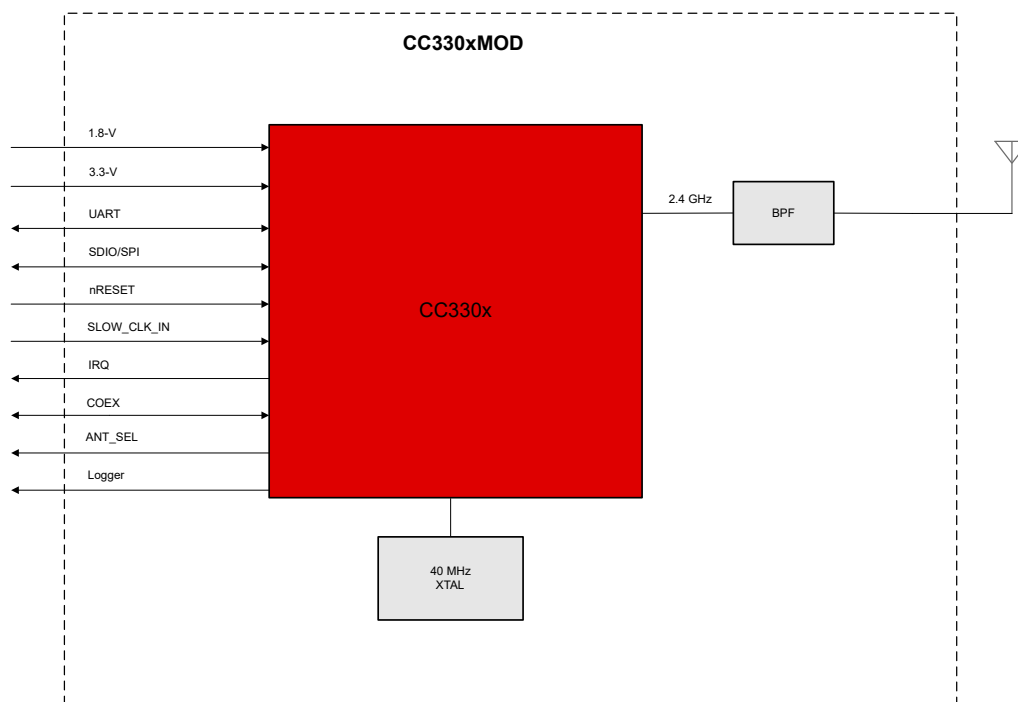
CC330xMOD のブロック図
