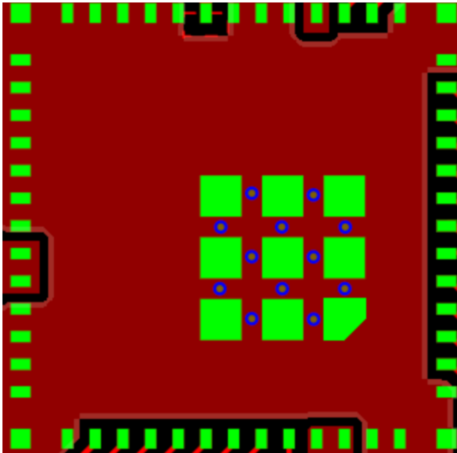
図 8-3. パッケージの底面にあるグラウンド パッドのブロック
