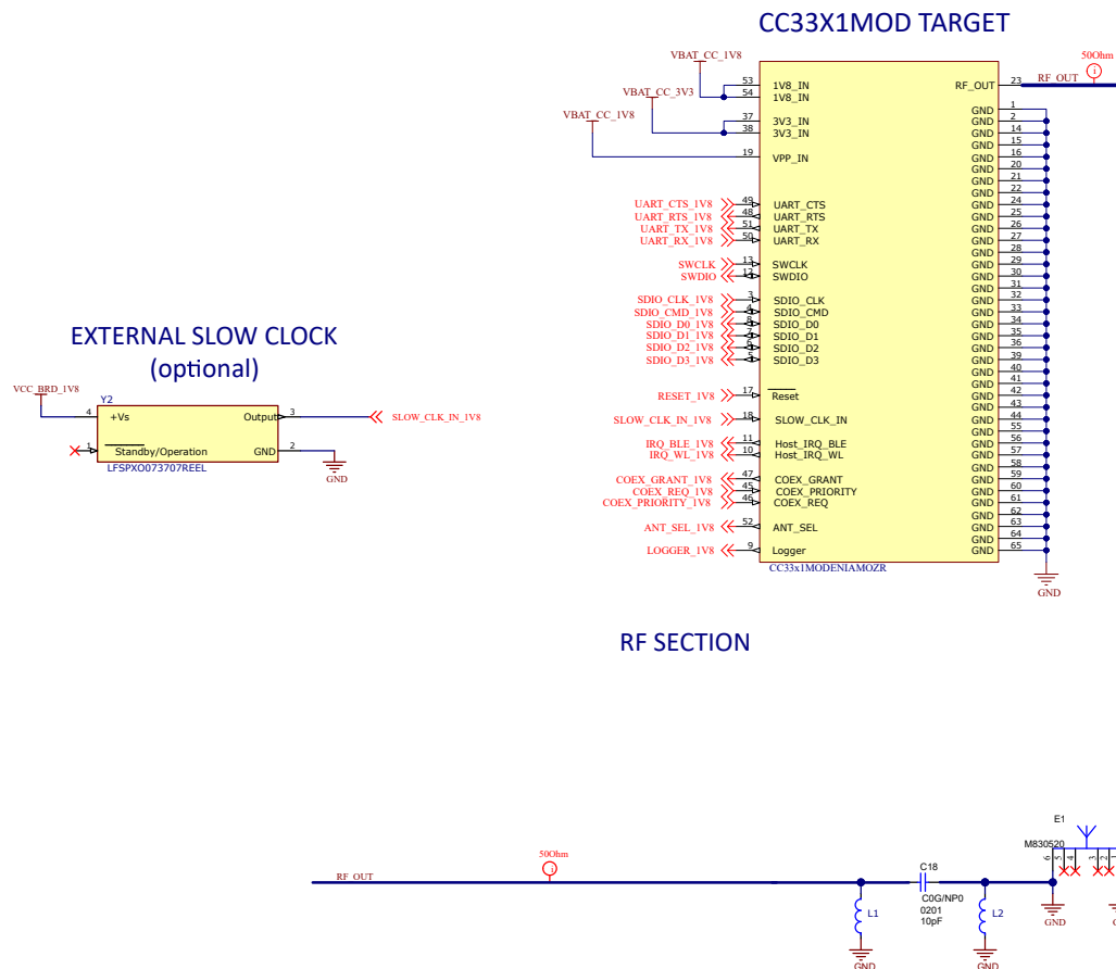
図 8-1. CC330xMOD のリファレンス回路図
