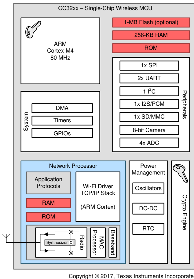
図 4-4. CC3220x ハードウェアの概要
