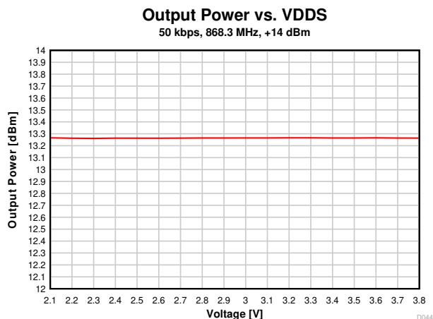
図 7-23. 出力電力と電源電圧との関係 (VDD5) (50kbps、868.3MHz)
