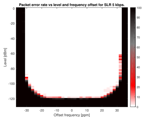
図 7-18. PER とレベルと周波数の関係 (SimpleLink™、長距離 5kbps、868MHz)
