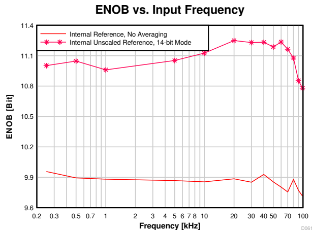
図 7-28. ENOB と入力周波数との関係
