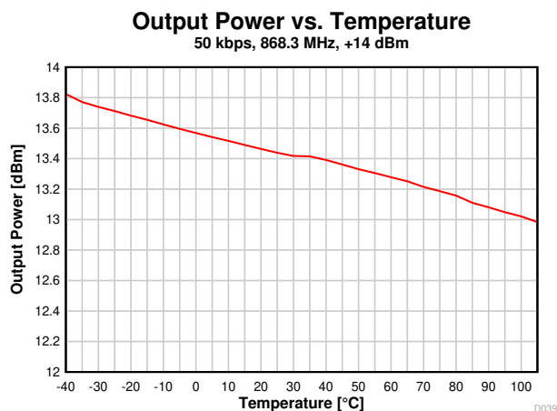
図 7-21. 出力電力と温度との関係 (50kbps、868.3MHz)
