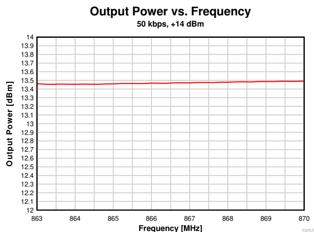
図 7-25. 出力電力と周波数との関係 (50kbps、868MHz)
