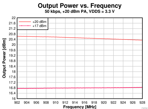
図 7-27. 出力電力と周波数との関係 (50kbps、915MHz、VDDS = 3.3V)
