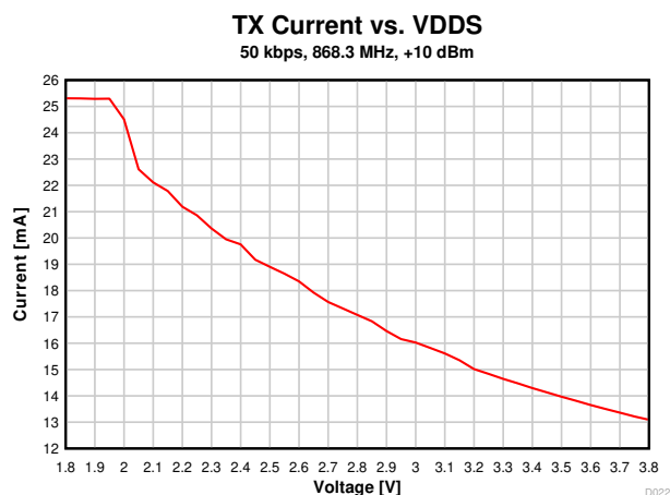
図 7-11. TX 電流と電源電圧との関係 (VDD5) (50kbps、868.3MHz)
