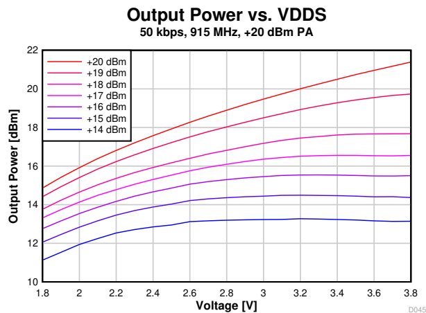
図 7-24. 出力電力と電源電圧との関係 (VDD5) (50kbps、915MHz)
