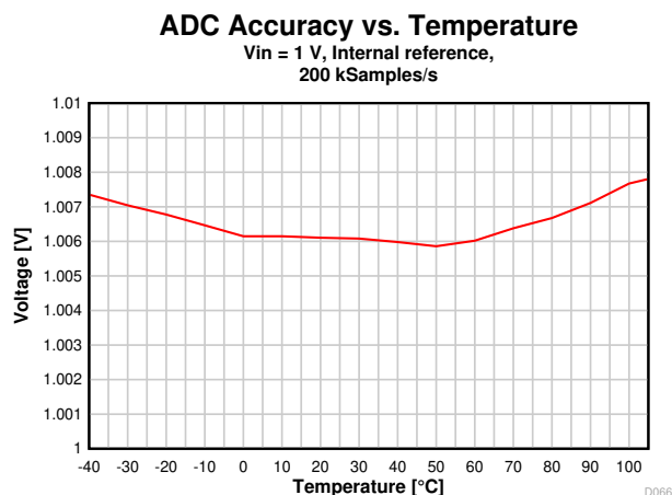
図 7-32. ADC の精度と温度との関係
