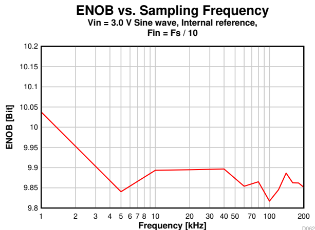
図 7-29. ENOB と サンプリング周波数との関係
