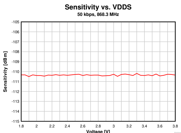
図 7-16. 感度と電源電圧との関係 (VDD) (50kbps、868.3MHz)
