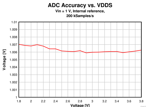
図 7-33. ADC の精度と電源電圧 (VDD) との関係
