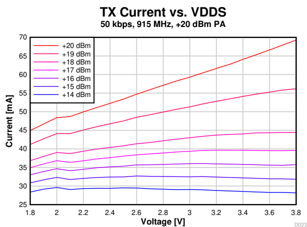
図 7-12. TX 電流と電源電圧との関係 (VDD5) (50kbps、915MHz)
