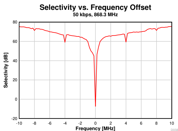
図 7-17. 選択性と周波数オフセットの関係 (50kbps、868.3MHz)
