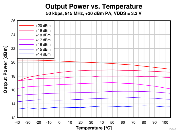
図 7-22. 出力電力と温度との関係 (50kbps、915MHz)
