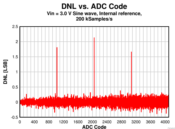
図 7-31. DNL と ADC コードとの関係
