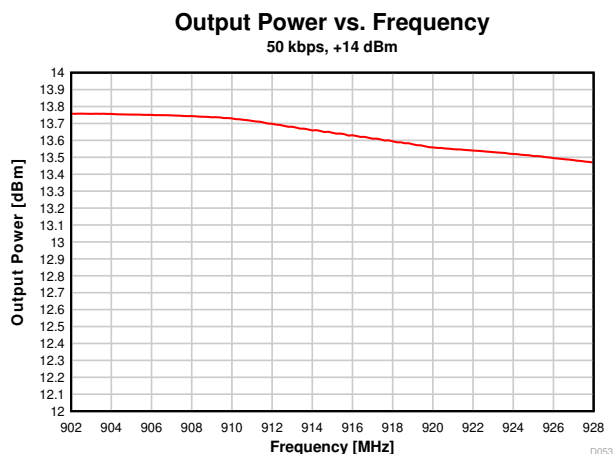
図 7-26. 出力電力と周波数との関係 (50kbps、915MHz)
