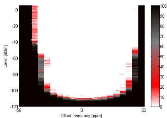
図 7-19. 802.15.4、50kbps、±25kHz の偏差、2-GFSK、100kHz の RX 帯域幅
