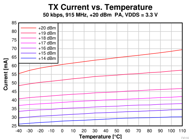
図 7-10. TX 電流と温度との関係 (50kbps、915MHz、VDD5 = 3.3V)
