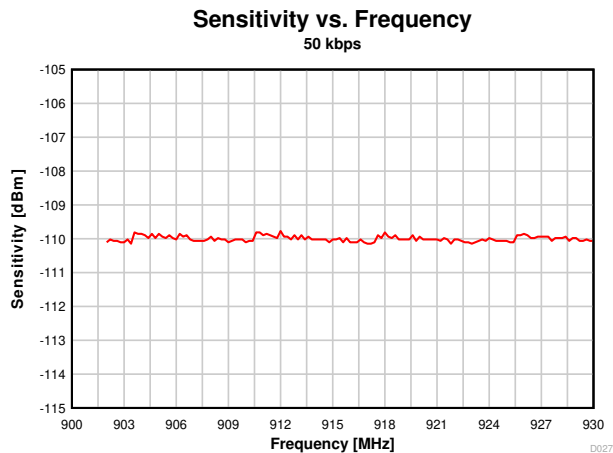
図 7-14. 感度と周波数との関係 (50kbps、915MHz)
