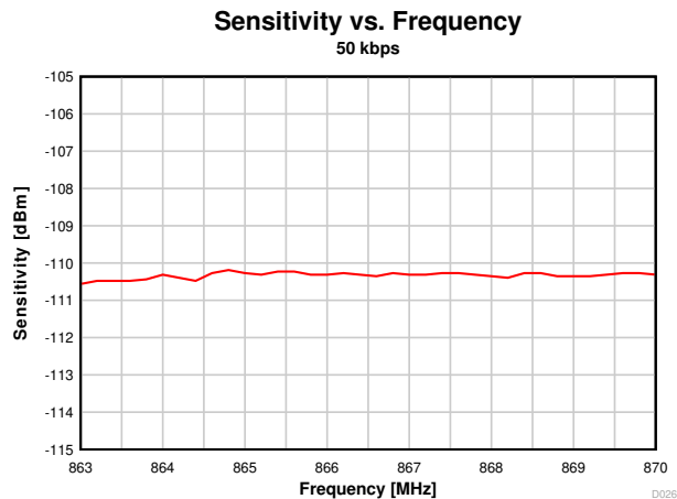
図 7-13. 感度と周波数との関係 (50kbps、868MHz)
