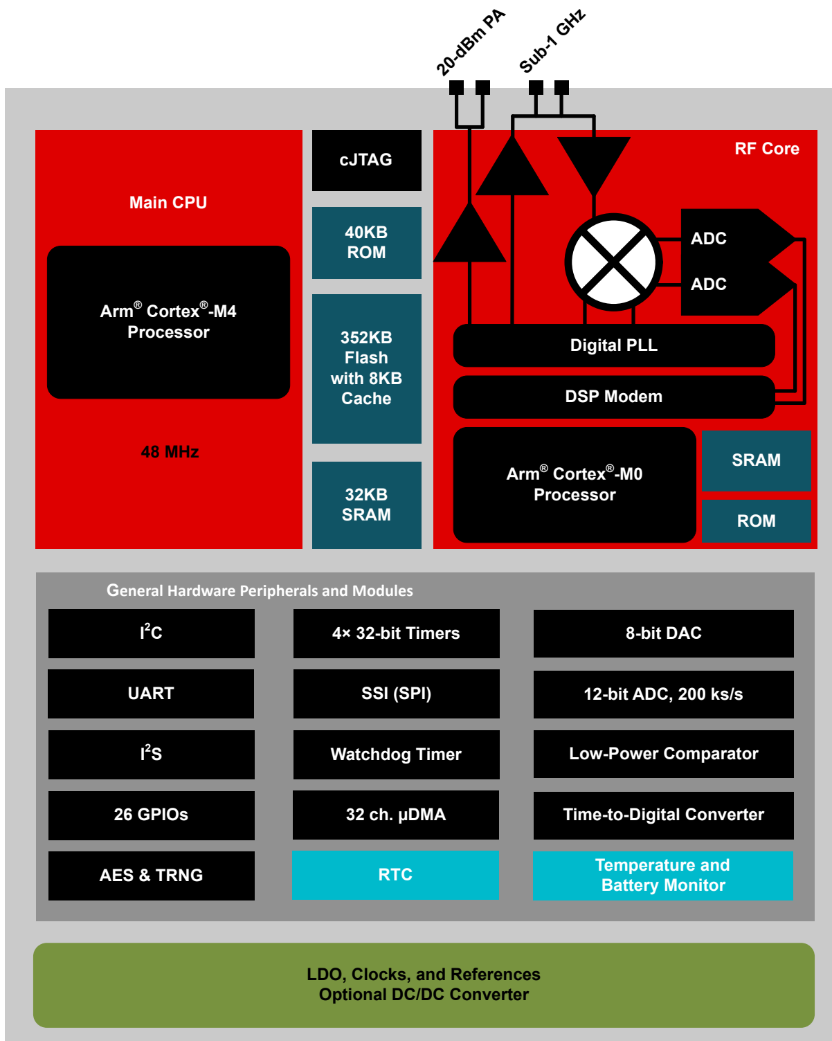
図 4-1. CC1311P3 機能ブロック図
