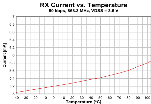
図 7-7. RX 電流と温度との関係 (50kbps、868.3MHz、VDD = 3.6)
