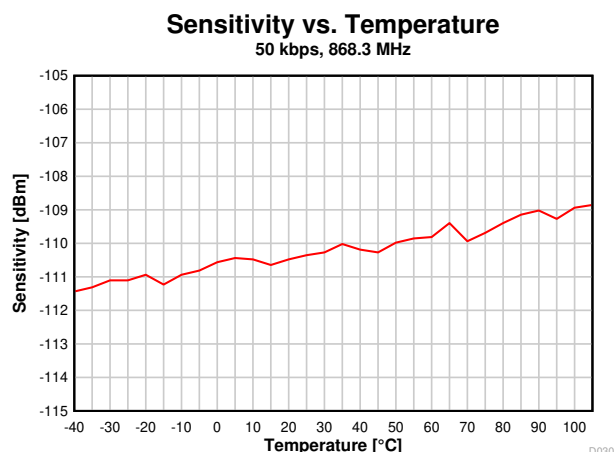
図 7-15. 感度と温度との関係 (50kbps、868.3MHz)
