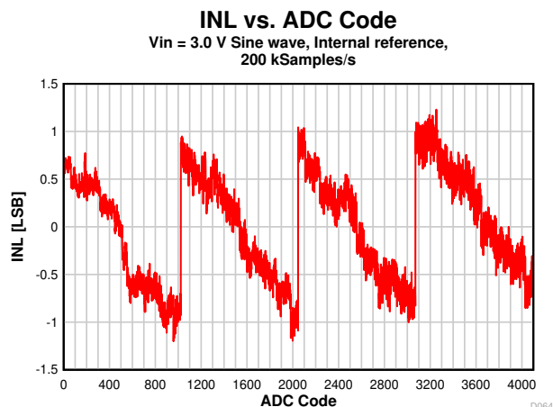
図 7-30. INL と ADC コードとの関係
