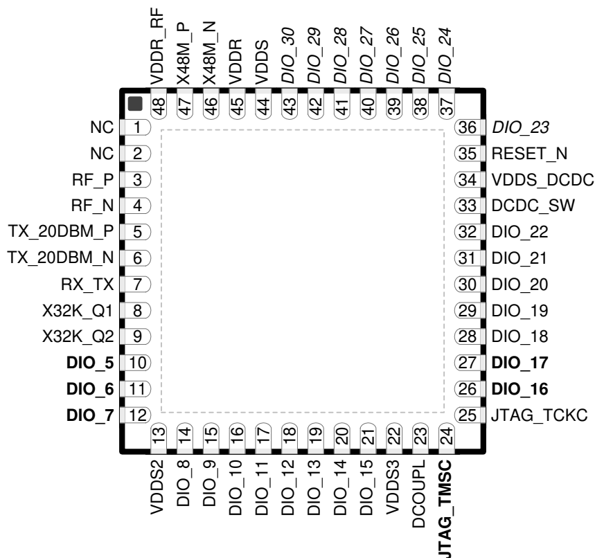
図 6-1. RGZ (7mm×7mm) ピン配置、0.5mm ピッチ (上面図)
