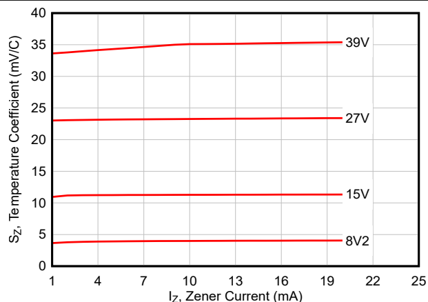
図 6-2. 温度係数
