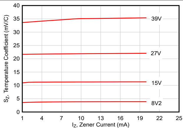
図 5-2. 温度係数
