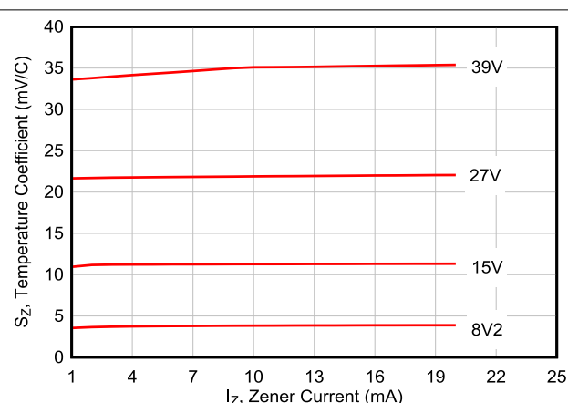
図 5-2. 温度係数
