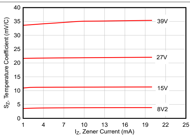
図 5-2. 温度係数
